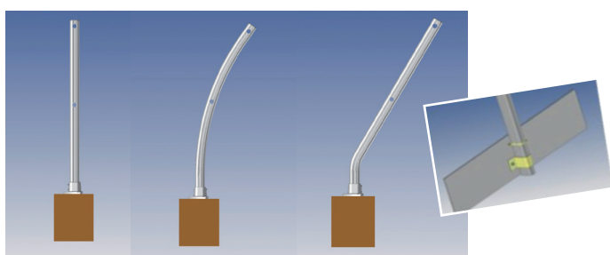
Poteaux sur fabrication en fonction de la hauteur d'acrotère
